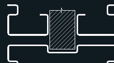
Συρόμενα εσωτερικά μονόφυλλης με σκοτία Interior, sliding, for single leaf door with recessed joint
