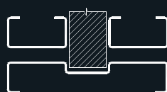
Συρόμενα εσωτερικά μονόφυλλης χωρίς σκοτία Interior, sliding, for single leaf door without recessed joint
