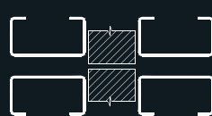
Συρόμενα εσωτερικά δίφυλλης χωρίς σκοτία Interior, sliding, for double leaf door without recessed joint
